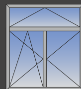
Δίφυλλο ανοιγόμενο - ανακλινόμενο με φεγγίτη
